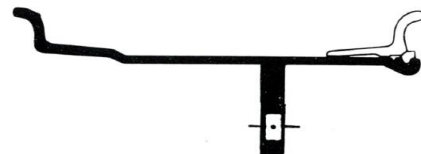
T Type Rim. Fixed Back Flange.
